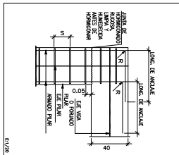
REINFORZAMIENTO DE PLATA DE BORDO CON VÍA Y FOLGADO
