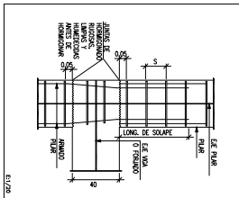
CAMPO DE CORTE DESPUÉS DE EL CAMPO DEL FOLGADO
